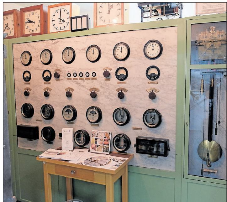
Kuban ist stolz, dass er diese Zentraluhr aus dem Stuttgarter Rathaus retten konnte. Sie zählt ebenfalls zu den besonderen Museumsstücken im Turmuhrenmagazin. Der Leiter braucht jedoch mehr Platz und hofft auf weitere Räume im Hochbunker. Foto: Frey
