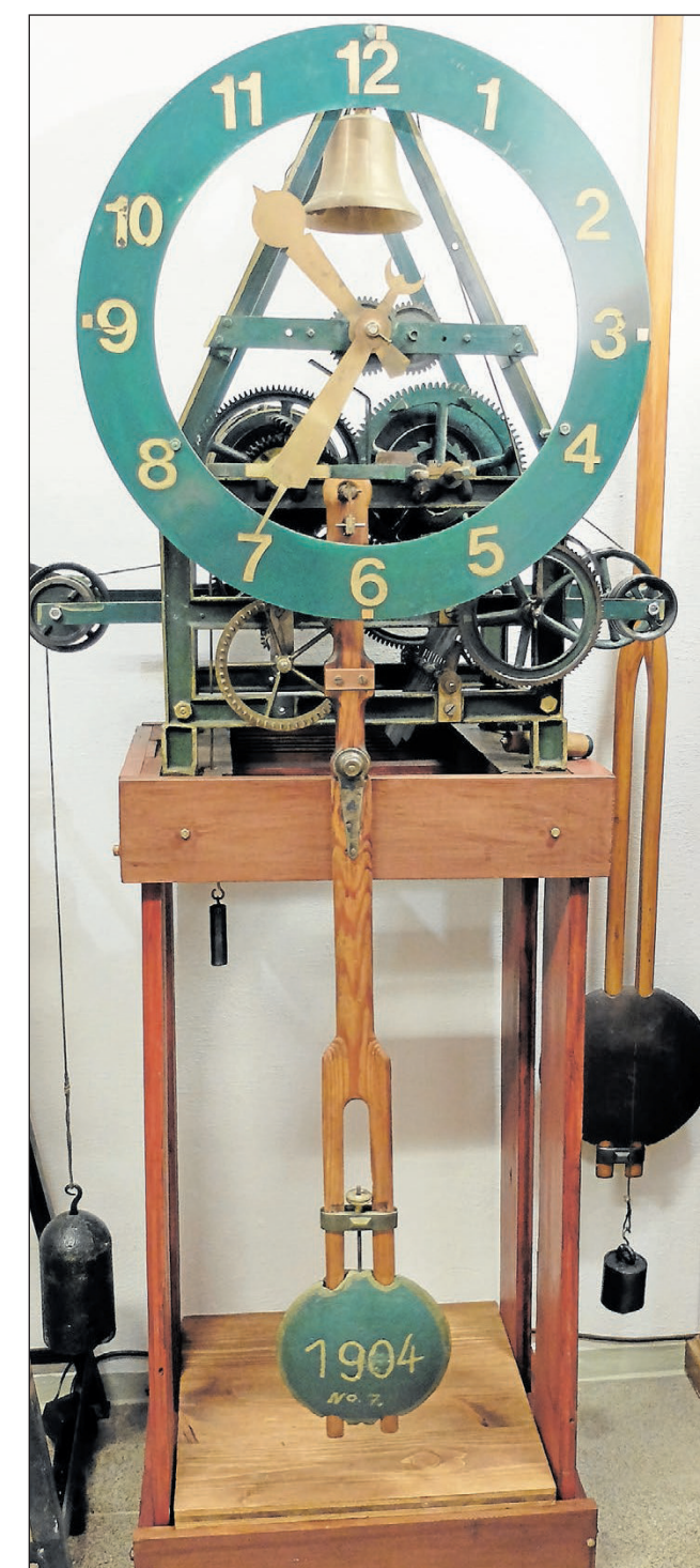
Ein Museumsstück: Eine Turmuhr aus dem Jahr 1904, die Kuban bis ins kleinste Detail aufwendig wieder restauriert und in Gang gesetzt hat.
